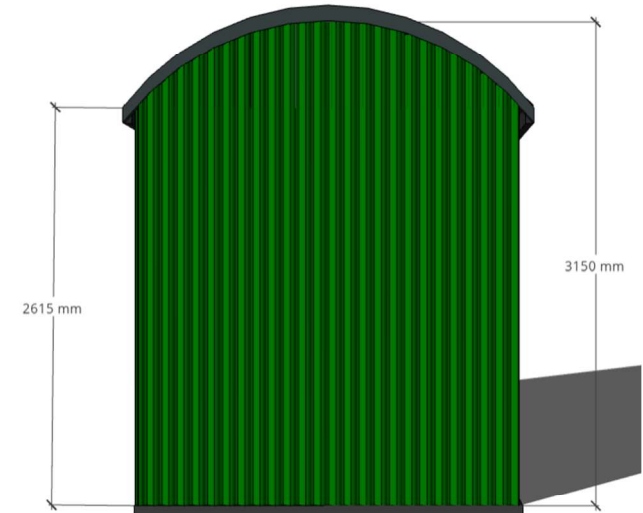
RHS ELEVATION
