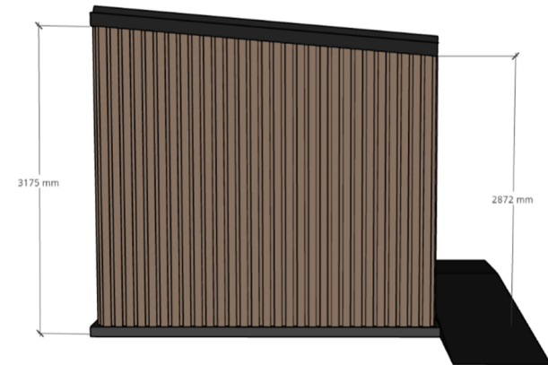
RHS ELEVATION
