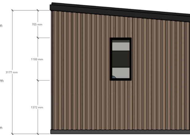
RHS ELEVATION
