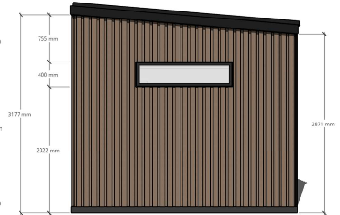
RHS ELEVATION
