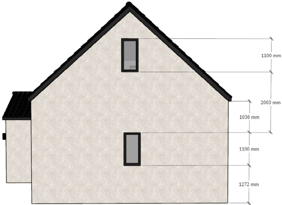
RHS ELEVATION
