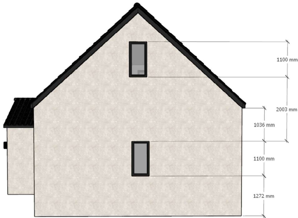
RHS ELEVATION
