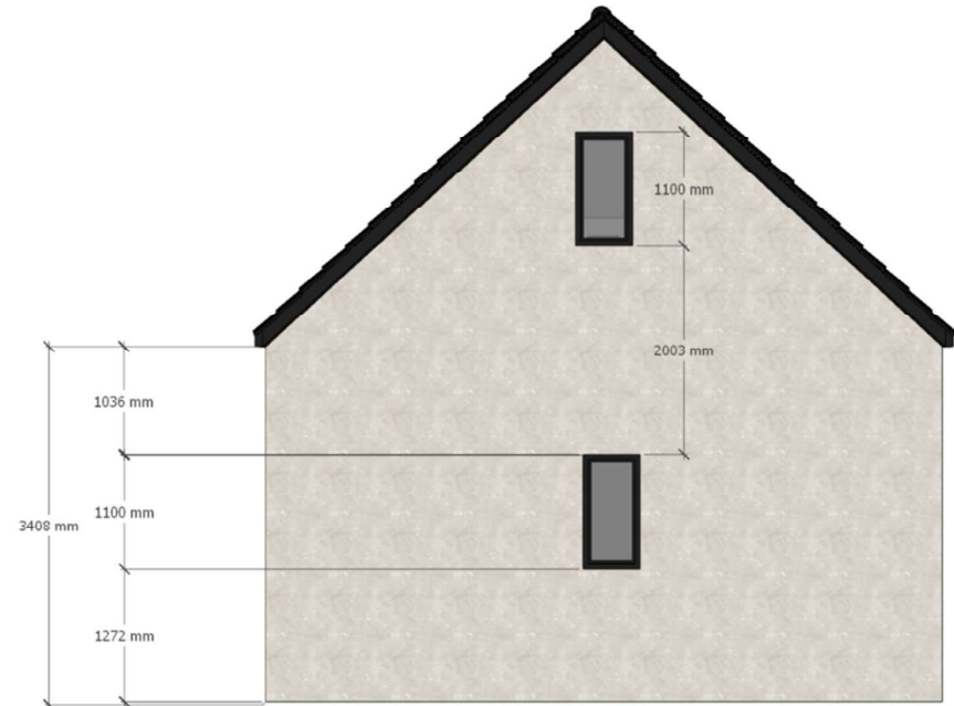
RHS ELEVATION
